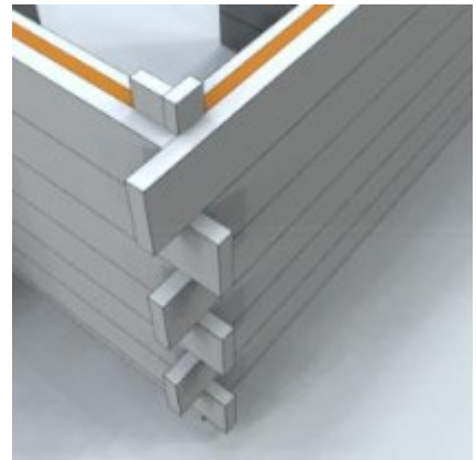
Detalle cruzado con aislante
