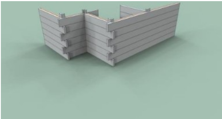
Opción rectangular cruzado con aislante
